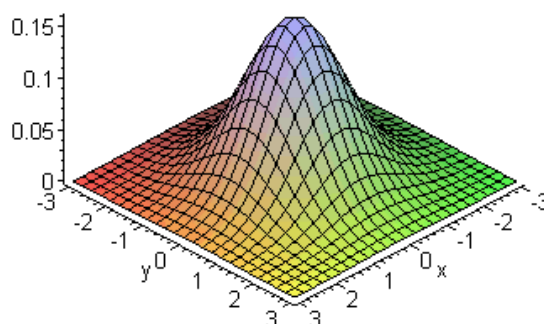
Рис. 3. Двумерная поверхность вероятности
